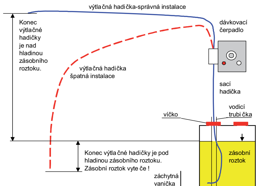
Obrázek č. 1: Příklad správné a špatné instalace dávkovacího čerpadla
