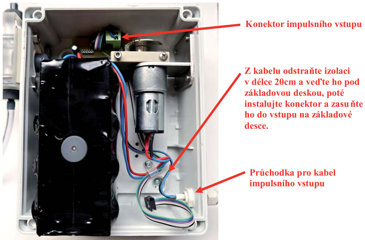
Obrázek č. 6: Dávkovací čerpadlo bez čelního panelu s popisky
